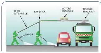
FIG. 1 - 2 SISTEMA SWEEPY JET
